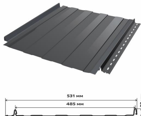
Трапеция
