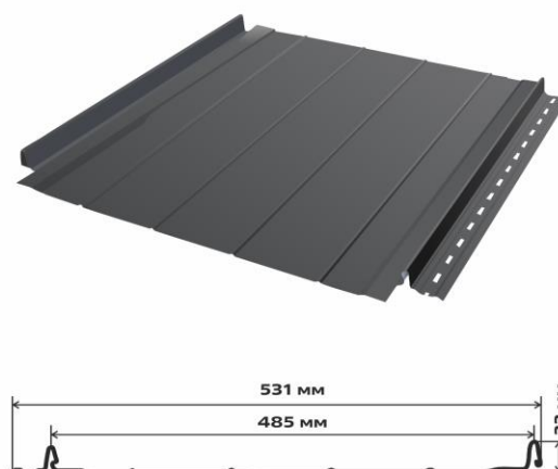
Накатка
