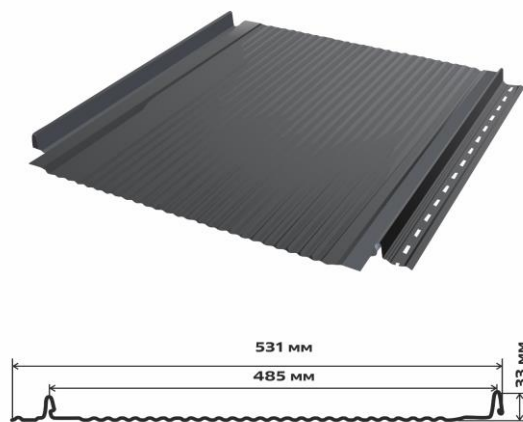
Накатка
