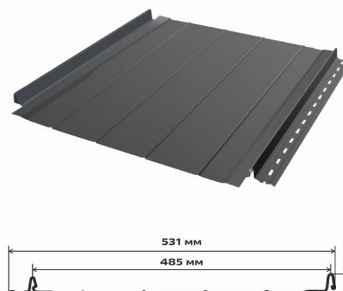
Накатка
