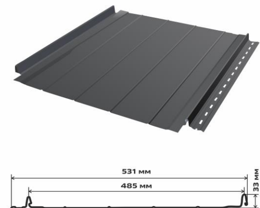
Накатка
